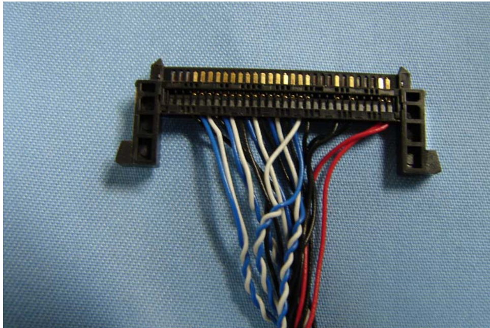
Foto 5. 3. Conector JAE
